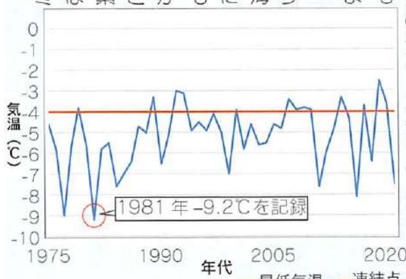
1975年(昭和50年)～2021年(令和3年)の最低気温推移
